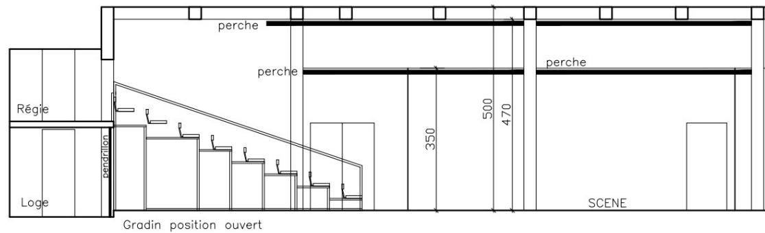
COUPE A-A'
