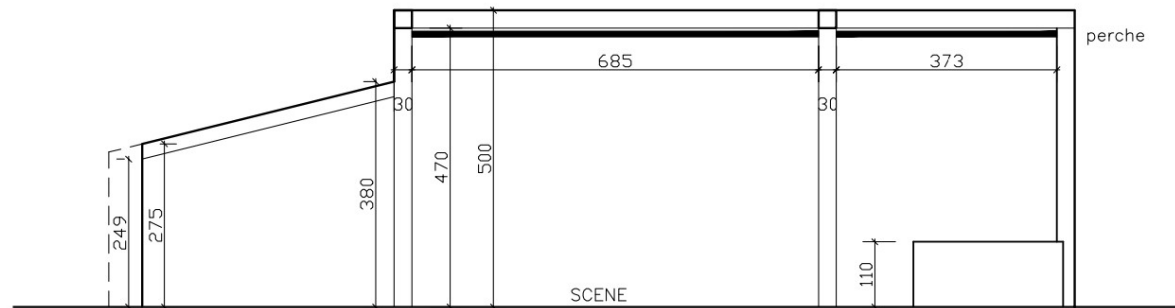
COUPE B-B'
